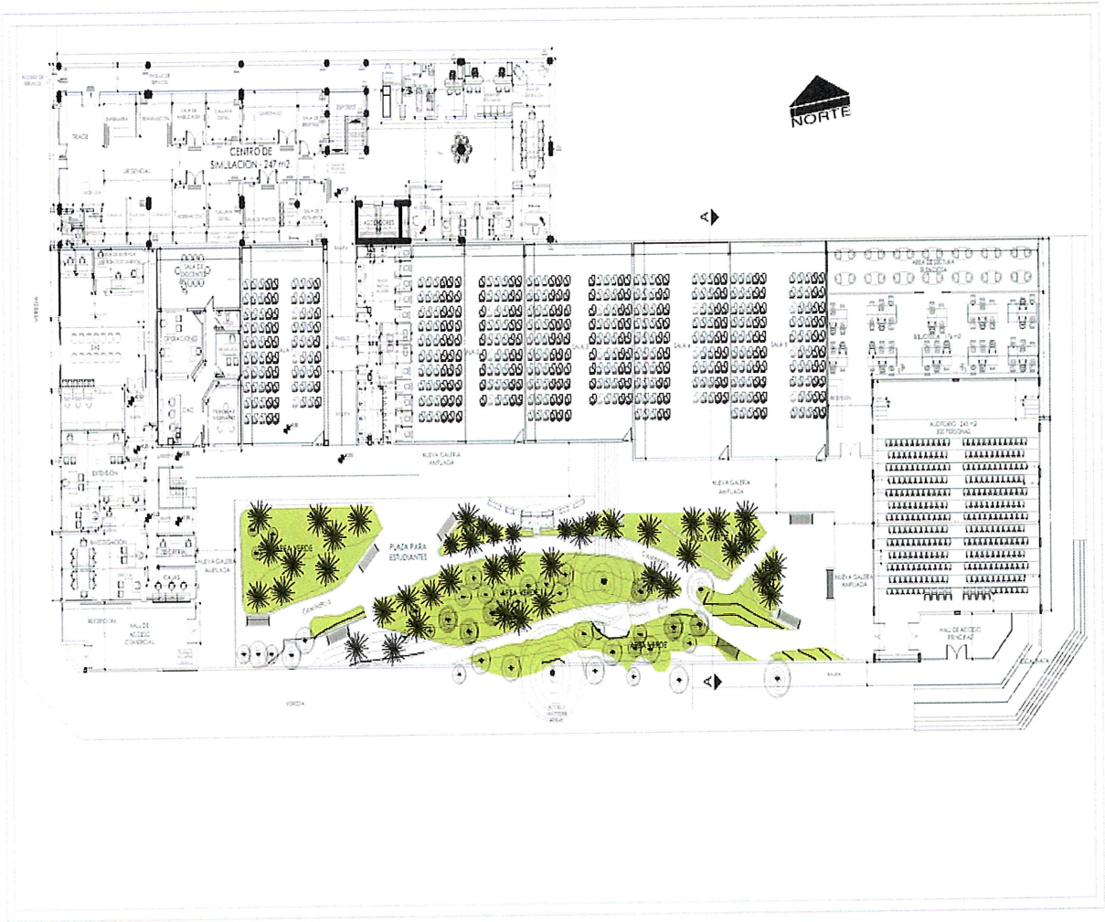
PLANTA BAJA - MASTER PLAN SEDE 1 - SDG ESC.: 1:100
